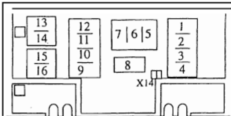
Schemat połączeń ścieżek przewodzących w modelu EZ-240
